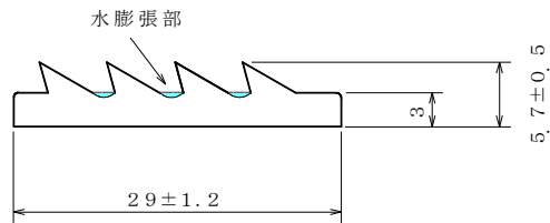
ゴム輪詳細図
