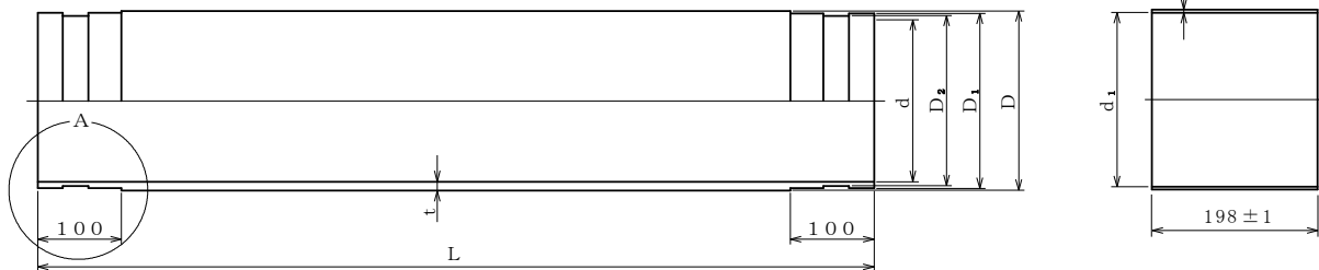
SUSカラー詳細図
