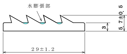
ゴム輪詳細図
